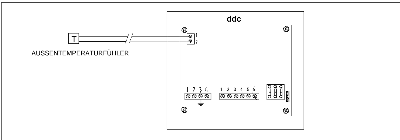
Abbildung 31 – ANSCHLUSSBEISPIEL AUSSENTEMPATURFÜHLER FÜR BETRIEBSMODUS WFüh
