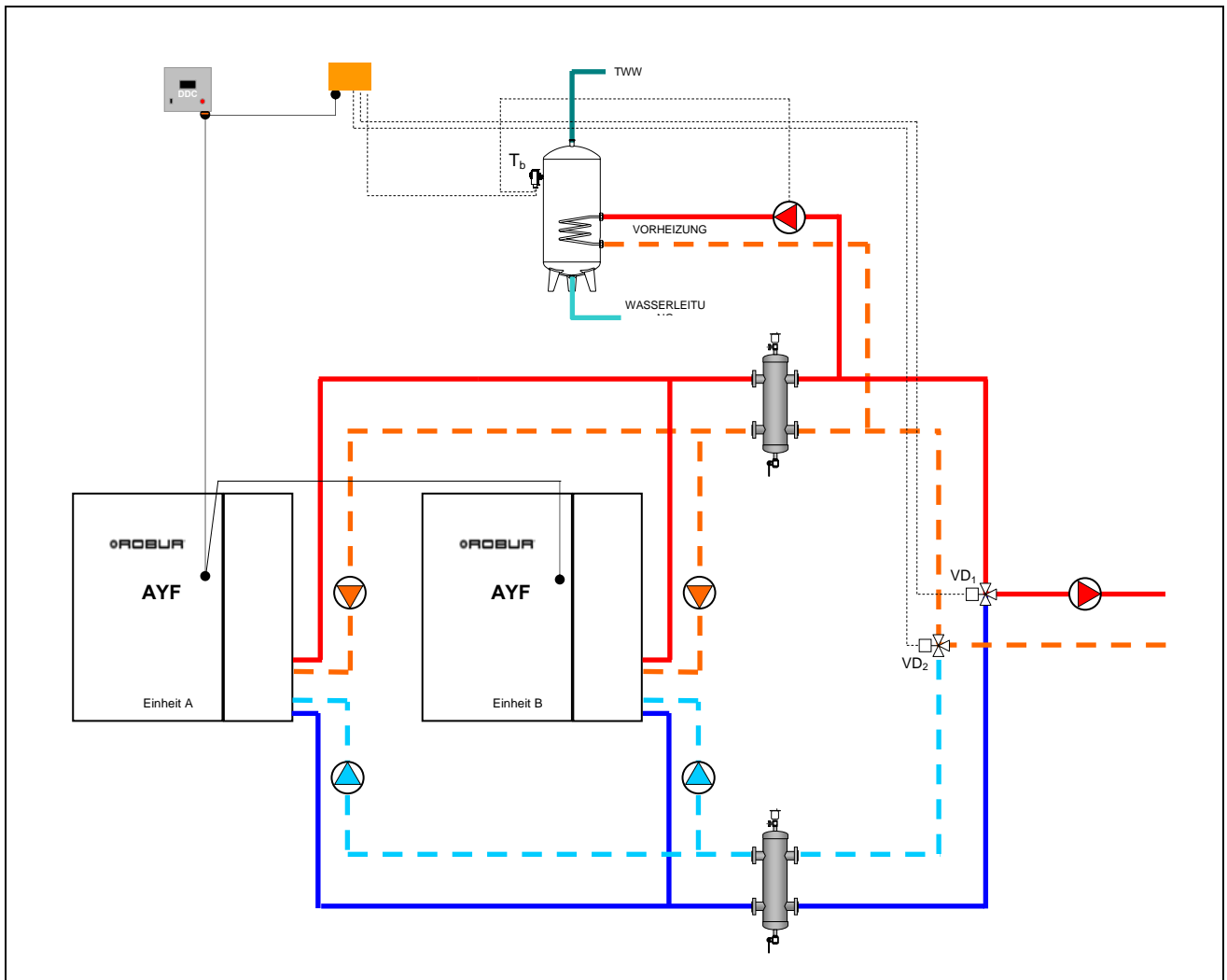
Abbildung 24 – VERWENDUNG TWW IM KÜHLBETRIEB
