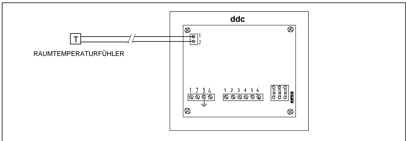
Abbildung 28 – ANSCHLUSSBEISPIEL RAUMTEMPERATURFÜHLER FÜR BETRIEBSMODUS RauT
