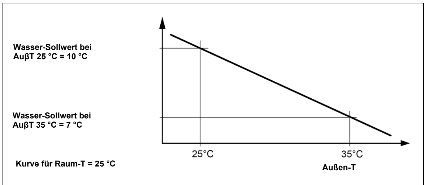
Abbildung 21 –DIAGRAMM DER "KÜHLKURVEN"
