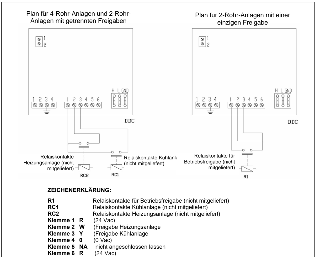
Abbildung 26 – BEISPIEL FÜR EINEN ANSCHLUSS EXTERNER KONTROLLSYSTEME IN BETRIEBSMODUS mRYW
