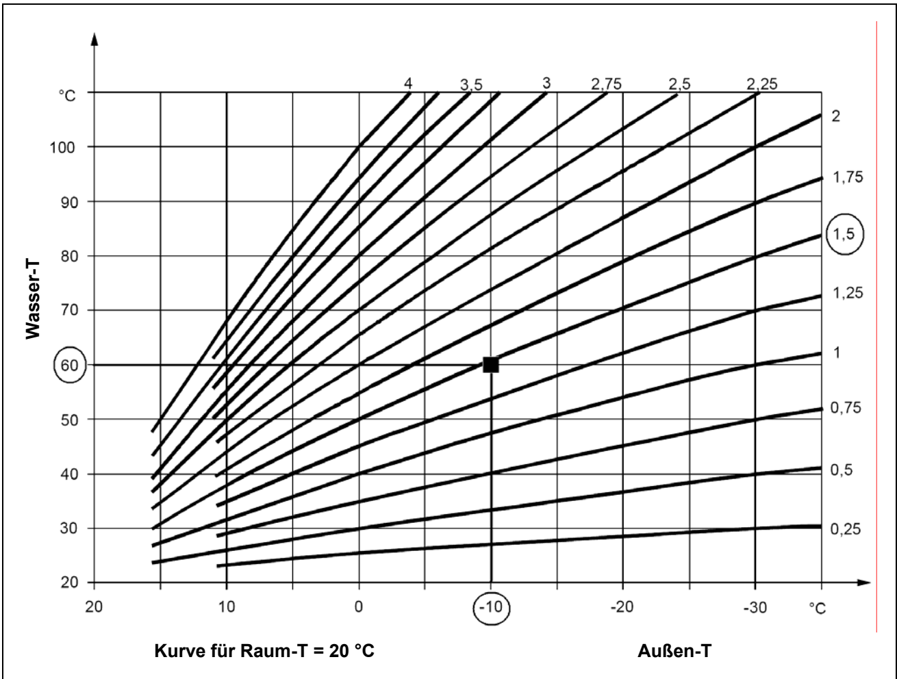
Abbildung 23 – BEISPIEL FÜR DIE WAHL EINER KURVE FÜR HEIZBETRIEB ENTSPRECHEND DER AUSLEGUNGSTEMPERATUR
