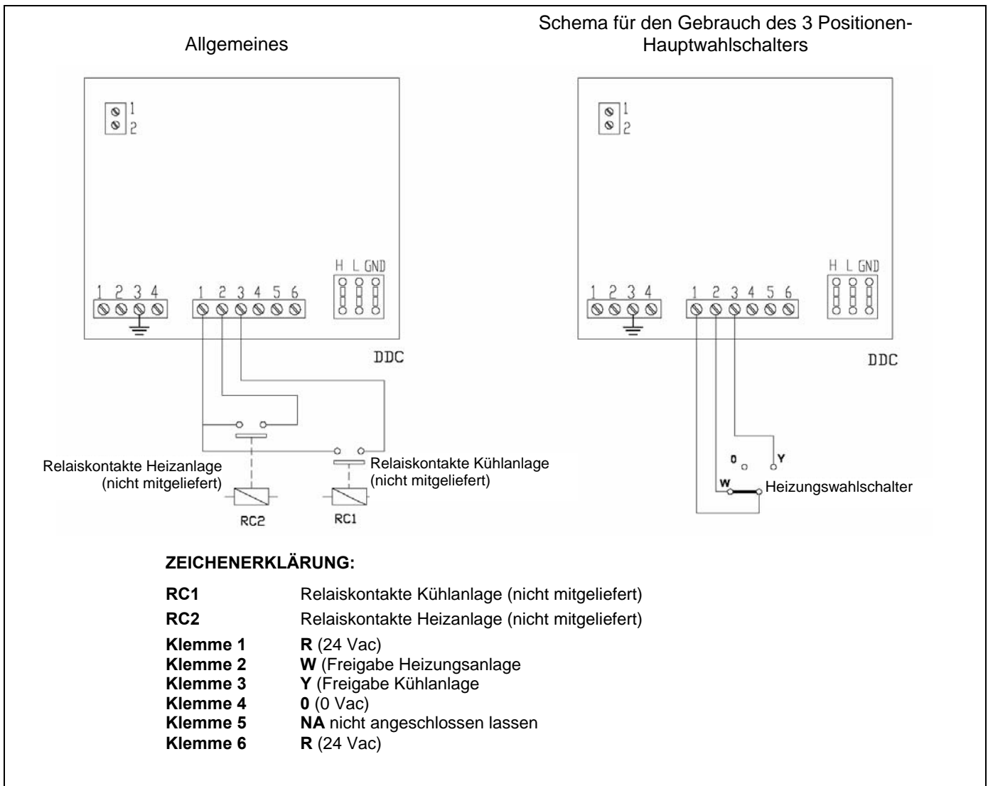
Abbildung 27 – BEISPIEL FÜR EINEN ANSCHLUSS EXTERNER KONTROLLSYSTEME IN BETRIEBSMODUS aRYW (NUR 2-ROHR-ANLAGEN)
