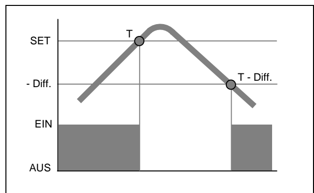
Abbildung 30 – FUNKTIONSPRINZIP BEI BETRIEBSMODUS RauT/AußT IN HEIZUNG
